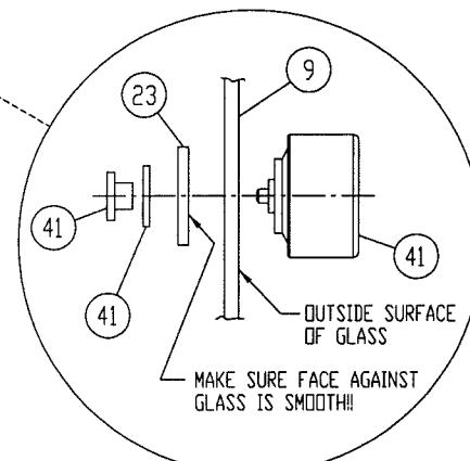
DOOR HOLD BACK STUD INSTALL 2X SCALE
